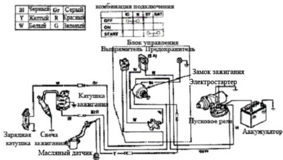
Электродиаграмма
