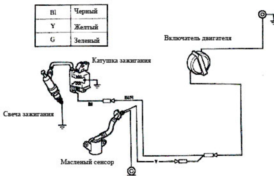
Электродиаграмма
